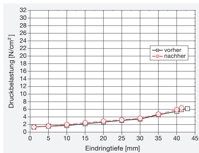
Bild 6: Verformbarkeit in Abhängigkeit vom Auflagedruck
